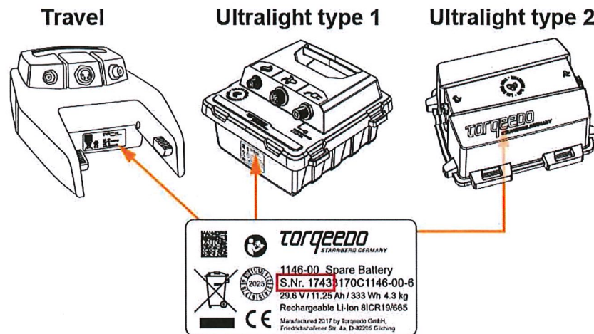
Abb.: Lage des Typenschildes mit Seriennummer
