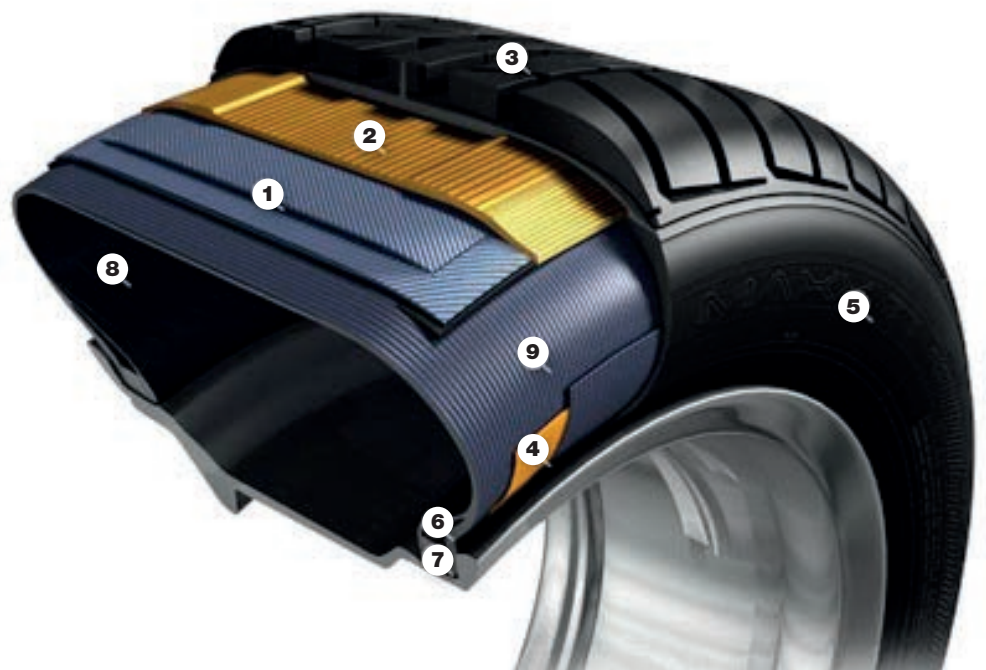
1 Stahlgürtel, 2 Abdecklage, 3 Laufstreifen, 4 Verstärkerstreifen, 5 Seitenwand, 6 Kernreiter, 7 Wulstkern, 8 Innerliner, 9 Karkasse. Quelle: Reifen24.de
